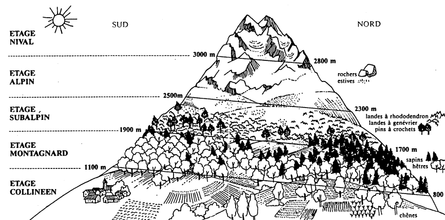
Les différents étages de végétation dans les Pyrénées avec leur végétation (d'après M. Gruber)
