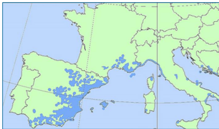
Aire naturelle de répartition d'une essence méditerranéenne : le Pin d'Alep
