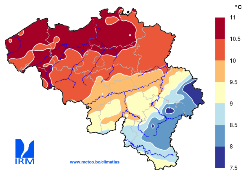
Températures moyennes annuelles en Belgique (Wallonie) Normales 1981 - 210
