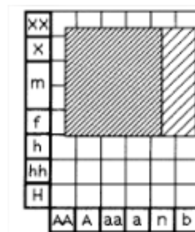
Ecogramme du Mélèze d'Europe
